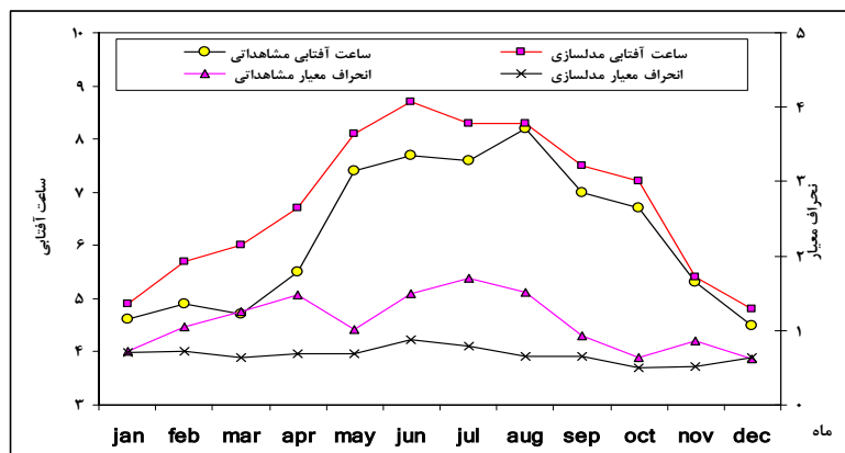
شکل (۱) نمودار میانگین‌های ماهانه مشاهده‌ای و شبیه‌سازی شده ساعت آفتابی و همچنین انحراف معیار آنها در ایستگاه گرگان (۲۰۰۷-۱۹۹۳)
