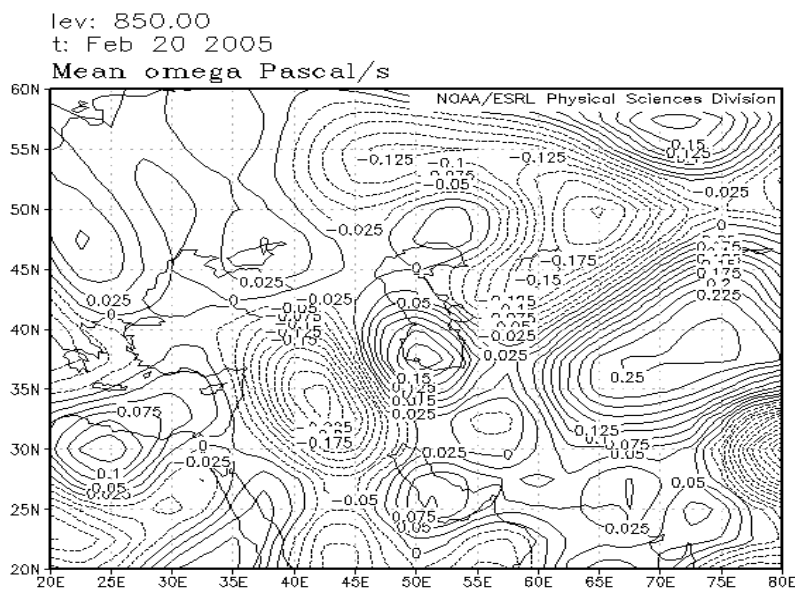
شکل (۲) نقشه امگای سطح ۸۵۰ hpa
