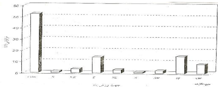
شکل ۷. هیستوگرام درصد فراوانی جهت وزش باد در جهت هشتگانه در ایستگاه قم
