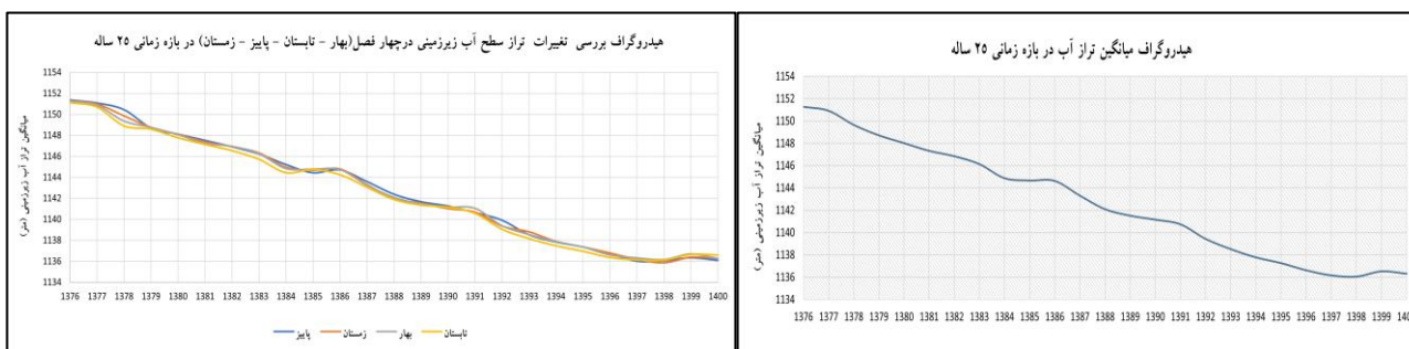
شکل (۲۰). هیدروگراف بررسی تغییرات تراز آب زیرزمینی در فصل بهار در بازه زمانی ۲۵ ساله (۱۴۰۰ - ۱۳۷۶)
