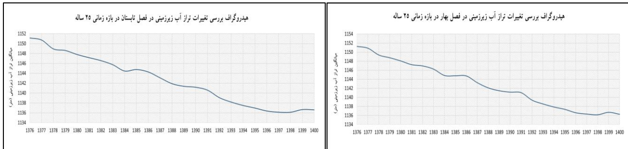
شکل (۱۶). هیدروگراف بررسی تغییرات تراز آب زیرزمینی در فصل تابستان در بازه زمانی ۲۵ ساله (۱۴۰۰ - ۱۳۷۶)
