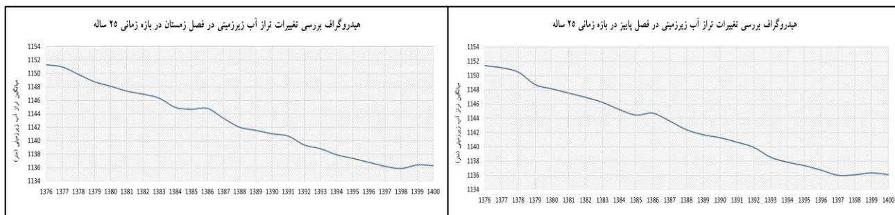
شکل (۱۸). هیدروگراف بررسی تغییرات تراز آب زیرزمینی در فصل زمستان در بازه زمانی ۲۵ ساله (۱۴۰۰ - ۱۳۷۶)
