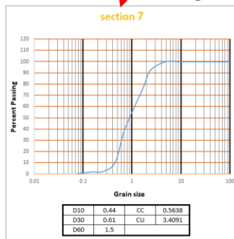
د- منحنی دانه‌بندی از نقطه ۷، بازه مکانی ۵
