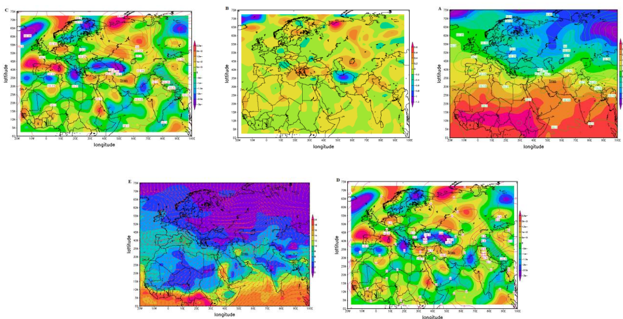
شکل (۶). (A): دمای (سلسیوس، ^{\circ}\text{C} ) و فشار (هکتوپاسکال، hpa) تراز دریا؛ (B): جبهه (کلون بر متر بر ثانیه و \text{ms}^{-1} ) تاوایی (متر بر ثانیه \text{ms}^{-1} ) و فشار (هکتوپاسکال، hpa) تراز دریا؛ (C): تاوایی (متر بر ثانیه \text{ms}^{-1} ) و فشار (هکتوپاسکال، hpa) تراز دریا؛ (D): تاوایی (متر بر ثانیه \text{ms}^{-1} ) و امگا (پاسکال بر ثانیه \text{Pa s}^{-1} ) تراز دریا؛ (E): باد مداری و نصف‌النهاری و شار همگرایی رطوبت (گرم بر کیلوگرم \text{g/kg} ) تراز دریا.
