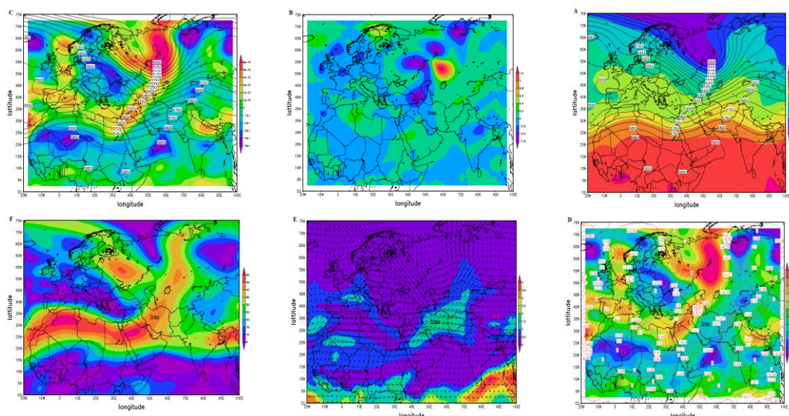
شکل (۹). (A): دما (سلسیوس، °C) و ارتفاع (ژئوپتانسیل متر) تراز ۵۰۰؛ (B): جبهه تراز ۵۰۰ هکتوپاسکال (کلون بر متر بر ثانیه 10^{-1} \times ms^{-1} ؛ (C): تاوایی (متر بر ثانیه ms^{-1} ) و فشار تراز ۵۰۰ هکتوپاسکال؛ (D): تاوایی و امگا (پاسکال بر ثانیه Pa s^{-1} ) تراز ۵۰۰ هکتوپاسکال و (E): باد مداری و شار همگرایی رطوبت (گرم بر کیلوگرم g/kg ) تراز ۵۰۰؛ (F): جت تراز ۳۰۰ هکتوپاسکال (متر بر ثانیه m/s ).
