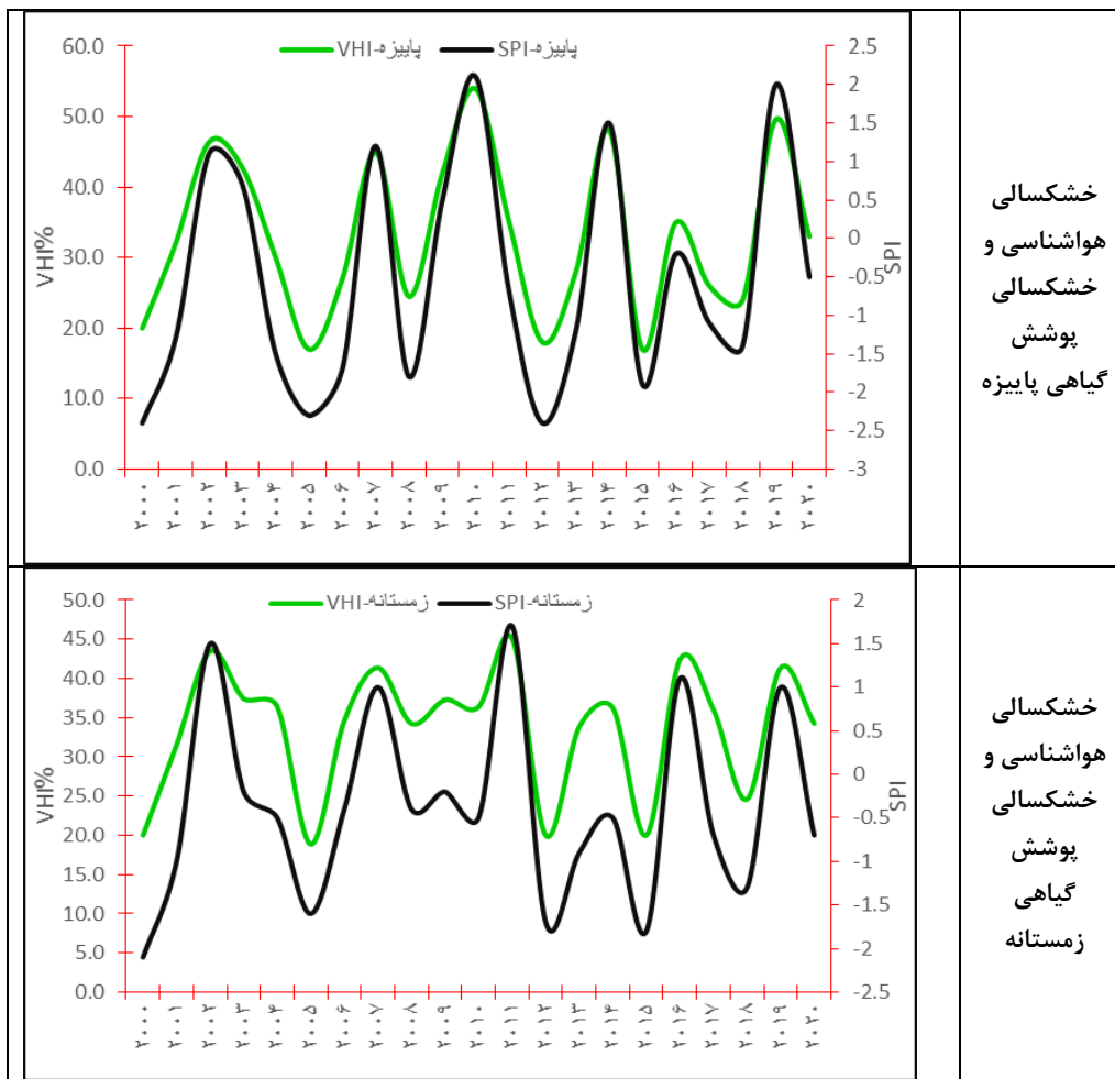
شکل (۲). روند سری زمانی شاخص‌های خشکسالی گیاهی VHI برای میانگین فضایی استان خوزستان و شاخص خشکسالی هواشناسی SPI براساس میانگین ایستگاه‌های سینوپتیک استان خوزستان در مقیاس فصلی طی دوره آماری ۲۰۰۰-۲۰۲۰
