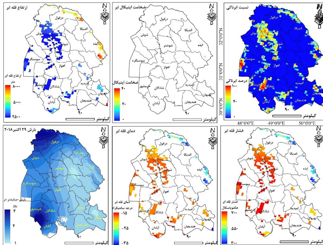
شکل (۴). پارامترهای ساختار میکروفیزیکی ابرهای مولد بارش متوسط ۲۹ اکتبر ۲۰۱۸ در سطح استان خوزستان (مستخرج از محصول MOD06 سنجنده MODIS) - مورد بارش سبک
