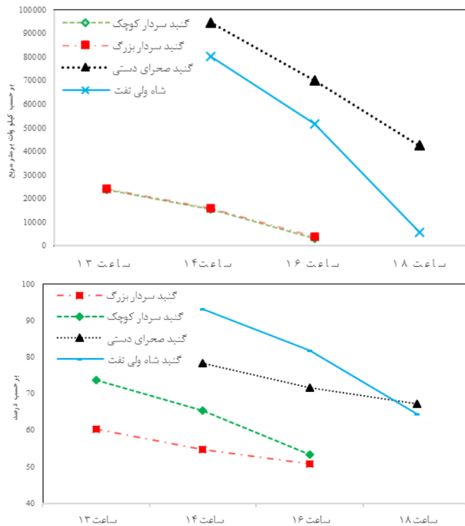
شکل (۹). از سمت بالا؛ نمودار دریافت تابش کل بر سطوح گنبدهای دهانه ثابت یزد و قزوین. از سمت پایین؛ نمودار درصد دریافت تابش بر سطوح گنبدها در ساعات ۱۳، ۱۴، ۱۶، ۱۸. منبع: نگارندگان.
