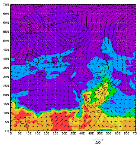
شکل (۴). وزش رطوبتی تراز ۸۵۰ هکتوپاسکال ۲۹ مارس ۱۹۹۷
