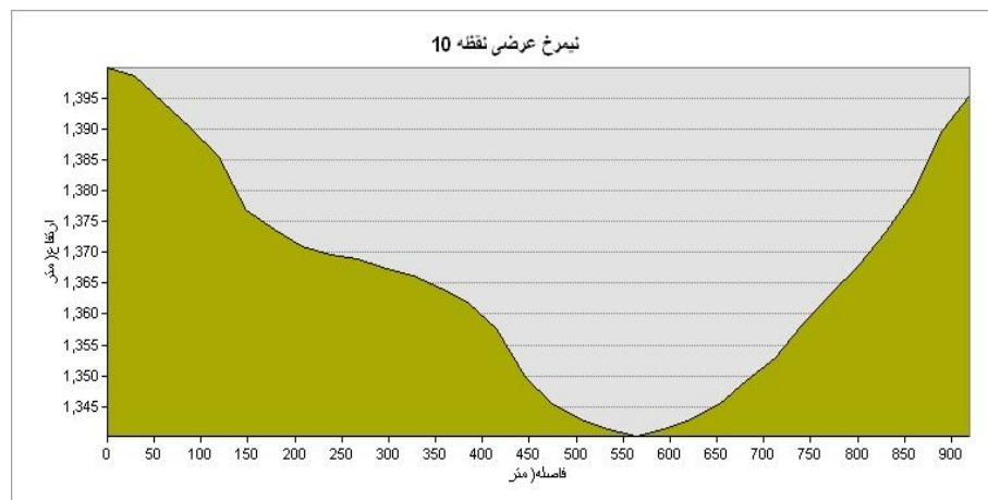
شكل (۸). نيمرخ عرضي در امتداد دره (منطقه بالادست، ميانه و پايين دست) رودخانه كن - سولقان
