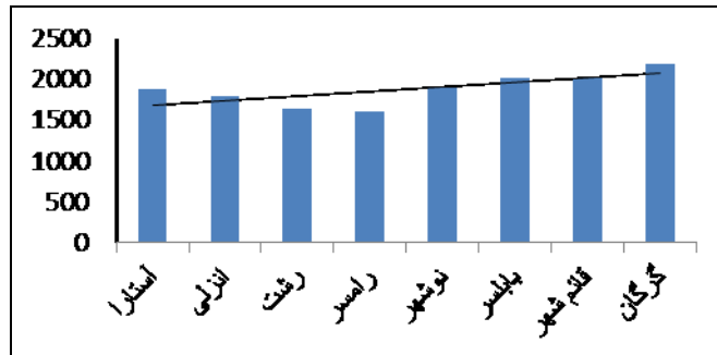
شکل (۶): نمودار ساعات آفتابی ایستگاه های منطقه
