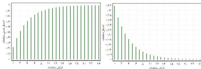
الف: نمودار تابع احتمال توزیع هندسی
