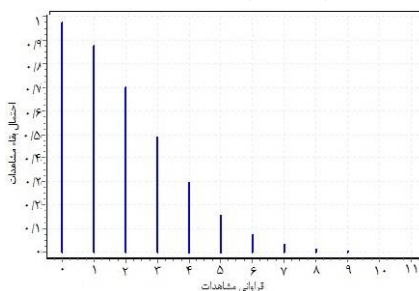
ج: نمودار تابع احتمال بقاء توزیع پواسون
