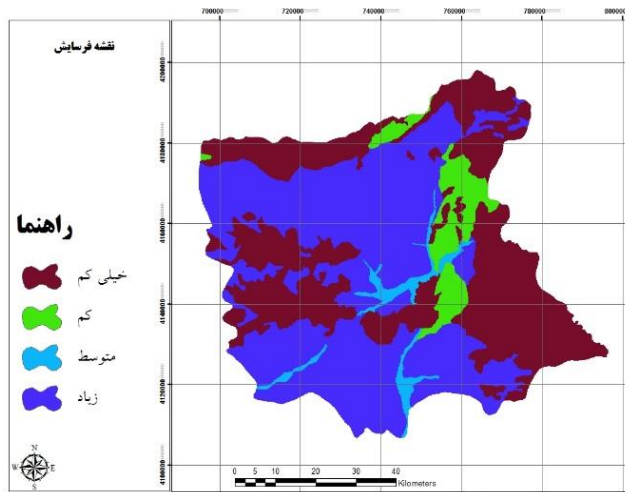
شکل (۱۳) فرسایش خاک
