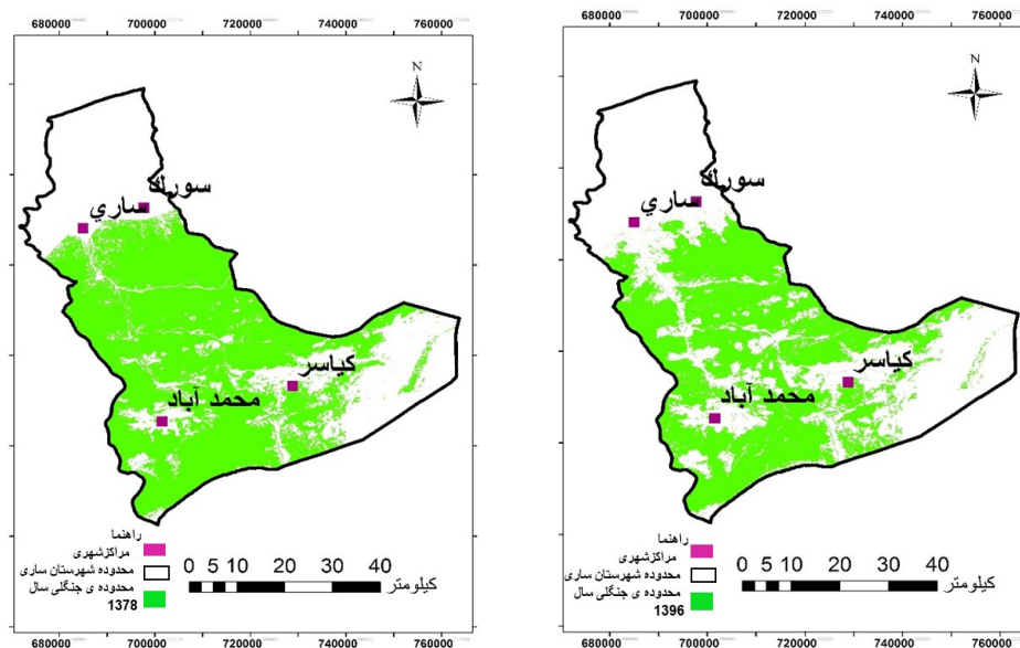
شکل (۲). نقشه جنگل و غیر جنگل مستخرج از تصویر TM برای سال 1378 (سمت چپ) نقشه جنگل و غیر جنگل مستخرج از تصویر OLI برای سال 1396 (سمت راست)
