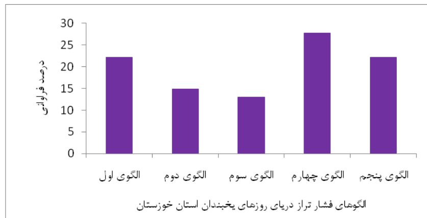
شکل (۱۳). درصد فراوانی هر یک از الگوهای فشار تراز دریا ی موجود یخبندان
