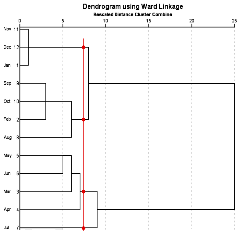
شکل (۱). دندروگرام (درخت خوشه‌بندی) ۴ خوشه‌ای حاصل از اعمال روش وارد بر فراوانی ماهانه وقوع روزهای توأم با توفان‌های گردوغباری ایستگاه خرم‌آباد
