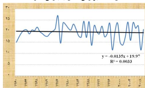
شکل (۱۳)، برازش مدل با بارش بهمن ماه
