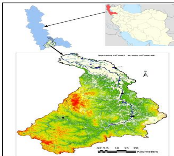
شکل(۱):حوضه آبریز سیمینه رود (نگارنده : دی ماه ۹۶)
