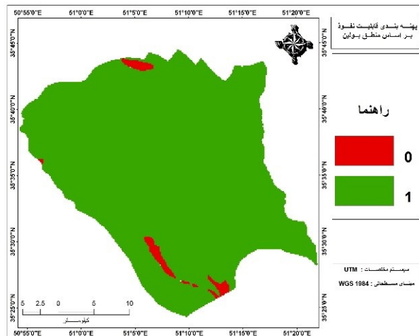
شکل(۱۳): نقشه وزنی طبقات مختلف قابليت نفوذپذيري
