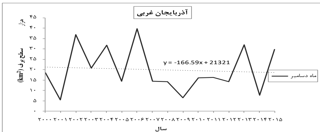
شکل ۹: تغییرات سطح برف در آذربایجان غربی طی سال‌های ۲۰۰۰ تا ۲۰۱۵ در ماه دسامبر با استفاده از داده‌های ماهواره‌ای مودیس
