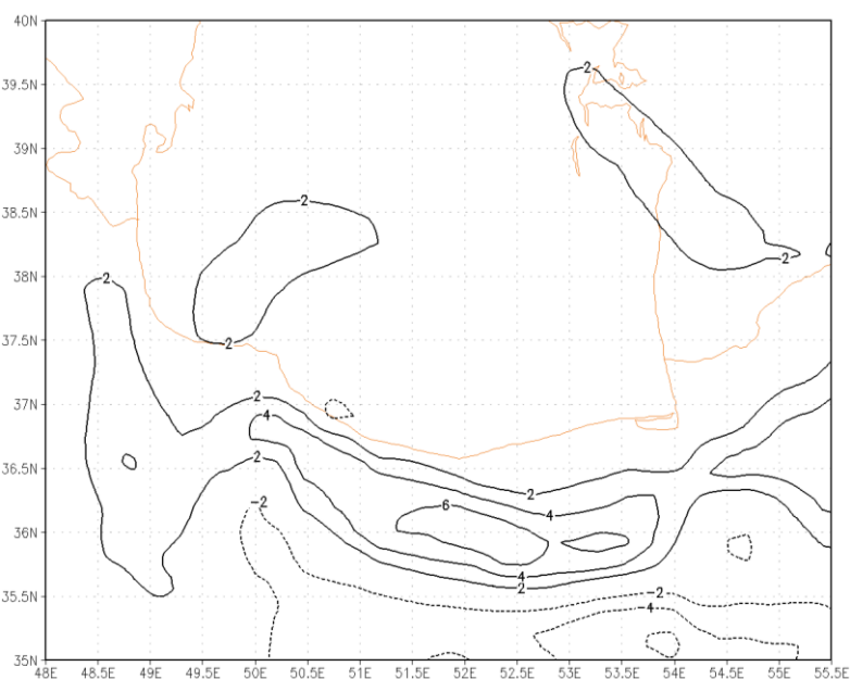
شکل (۴). تفاوت ماهانه دما سطح زمین به درجه سانتی‌گراد حاصل از تفاضل‌گیری بین شرایط حذف توپوگرافی و شرایط مرجع در ساعت ۱۲ GMT
