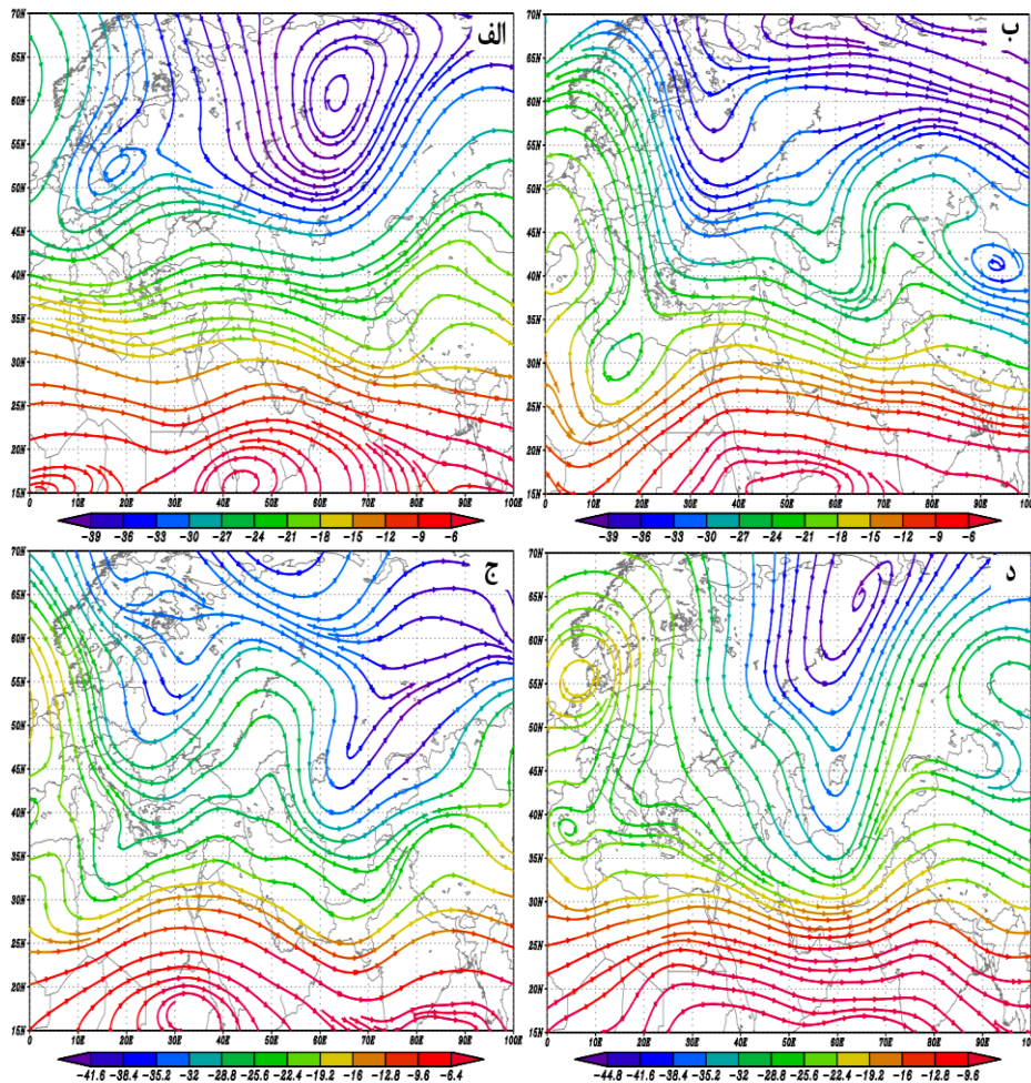
شکل (۵). نقشه های وزش دمایی تراز ۵۰۰ هکتوپاسکال (الف) روز ۱۲ دسامبر ۱۹۶۳ (طبقه امواج سرد ضعیف)، (ب) روز ۱۱ ژانویه ۱۹۶۳ (طبقه امواج سرد متوسط)، (ج) روز ۷ ژانویه ۱۹۶۴ (طبقه امواج سرد بسیار شدید)، (د) روز ۲۰ ژانویه ۱۹۶۴ (طبقه امواج ابر سرد).
