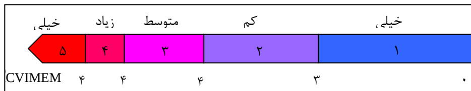
شکل (۳) طیف آسیب پذیری اقلیمی
