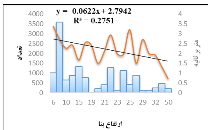
شکل (۱۴). نمودار ارتفاع ساختمان و سرعت باد منطقه یک
