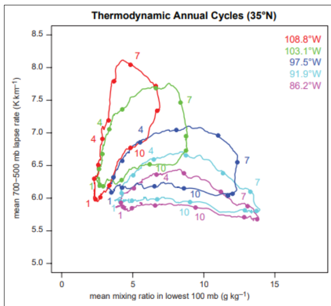
شکل (۱). چرخه سالانه آهنگ افت دمای لایه‌های میانی و رطوبت در ۷۰۰-۵۰۰ هکتوپاسکال
