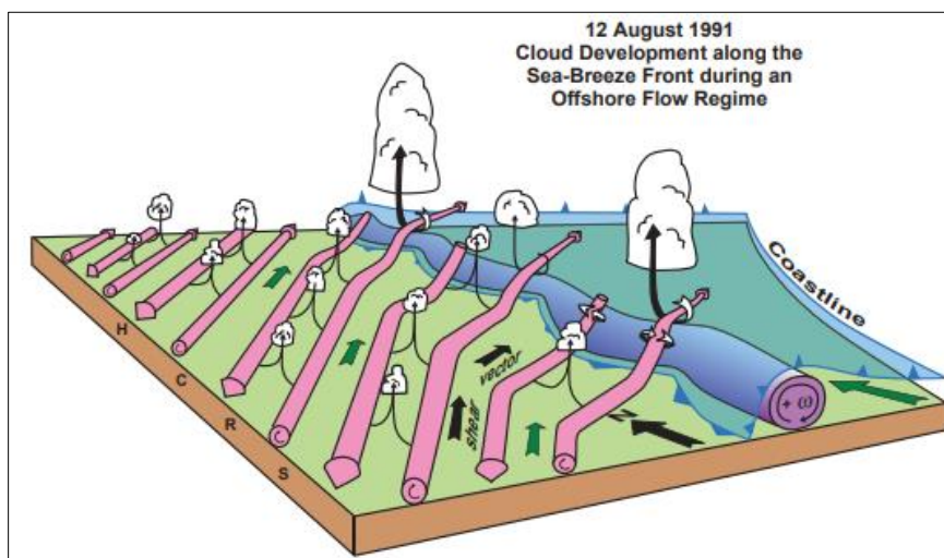
شکل (۱۱). شمایی از برهمکنش بین جبهه نسیم دریا و پیچک‌های همرفتی افقی و چگونگی ارتباط آن‌ها با شکل‌گیری توسعه شمایی از برهمکنش بین جبهه نسیم دریا و پیچک‌های همرفتی افقی و چگونگی ارتباط آن‌ها با شکل‌گیری توسعه ابر در ۱۲ آگوست ۱۹۹۱ در طی آزمون باردار شدن الکتریکی بارش همرفتی
