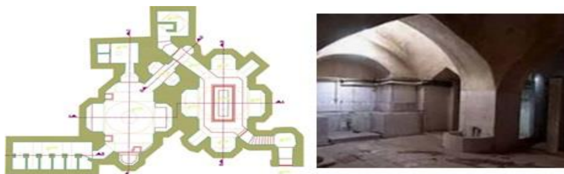
شکل (۱۲). پلان بینه و گرمخانه حمام میدان کنگاور (منبع: آرشو میراث فرهنگی استان کرمانشاه، ۱۳۹۹)
