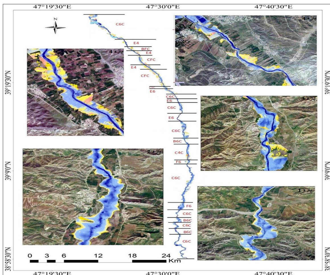
شکل (۵). طبقه‌بندی ژئومورفولوژیکی مجرای رودخانه دره ائورت بر اساس مدل رزگن
