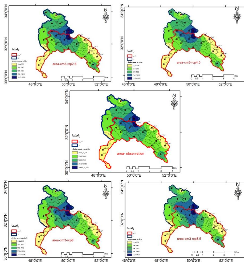
شکل (۴). مدل CM3 میانگین بارش آبی حوضه دز و کارون در طول دوره ۲۰۲۱-۲۰۵۰ نسبت به میانگین بارش مشاهداتی در طول دوره آماری ۱۹۷۶-۲۰۰۵)
