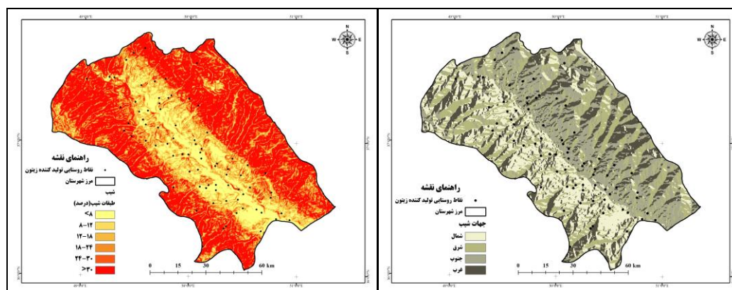
شکل (۸). پهنه‌بندی پارامتر جهت‌شیب
