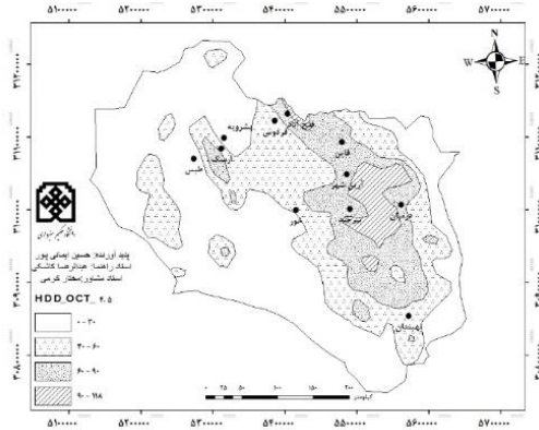
شکل (۸). پراکنش مکانی نیازهای گرمایشی مهر، دوره آینده (۲۰۱۶-۴۱) سناریو RCP_4.5
