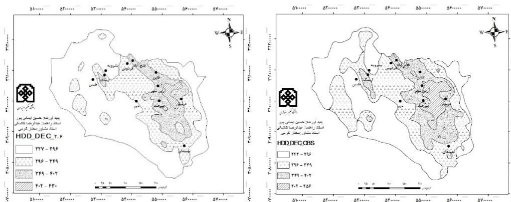
شکل (۱۴). پراکنش مکانی نیازهای گرمایشی آذر در دوره مشاهده ای (۱۹۹۰-۲۰۱۵) و شکل (۱۵). پراکنش مکانی نیازهای گرمایشی آذر در دوره
