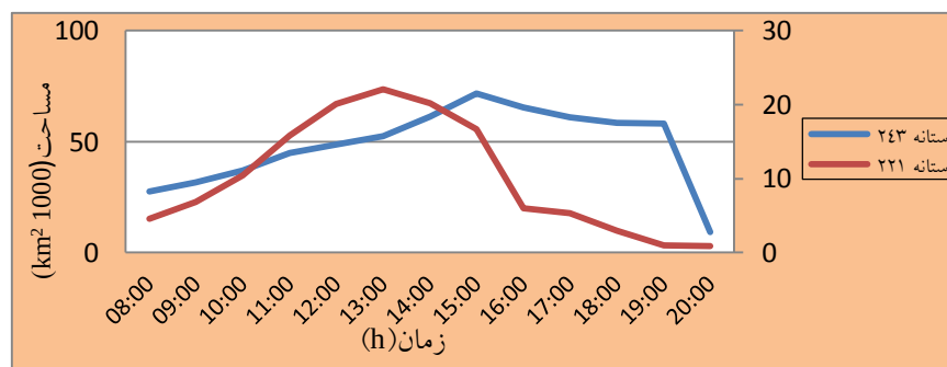
شکل (۲). مقایسه تغییرات مساحت سامانه‌های همرفتی میان‌مقیاس در دو آستانه ۲۴۳ و ۲۲۱ کلون
