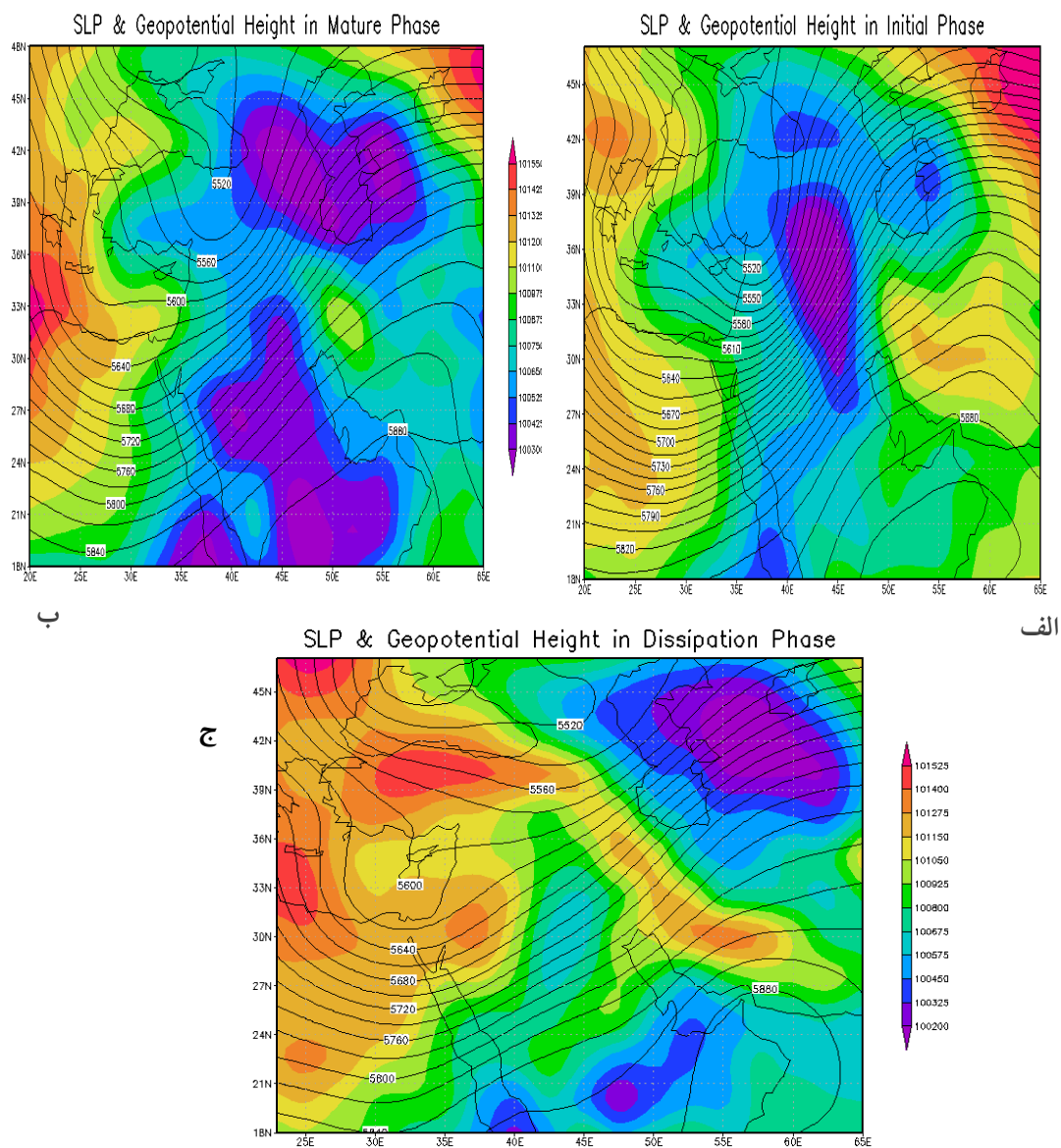
شکل (۸). نقشه‌های سطح زمین و ارتفاع ۵۰۰ هکتوپاسکال الف. شکل‌گیری ب. بلوغ ج. زوال
