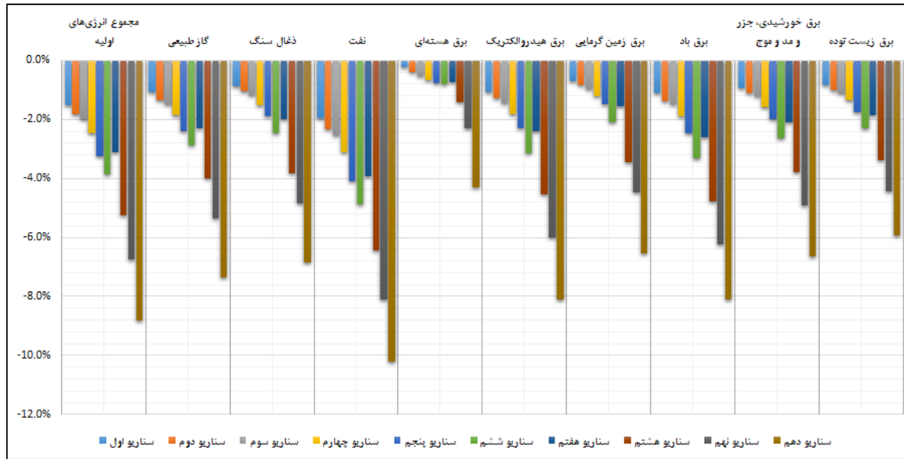
نمودار ۱. تغییرات مصرف انرژی‌های اولیه در منطقه منا
