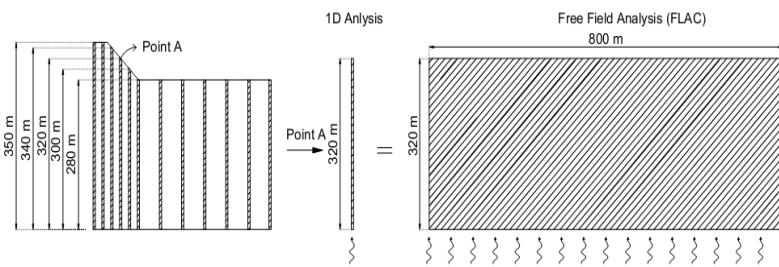
شکل ۴. مدل میدان آزاد در نرم‌افزار FLAC_{2D}
