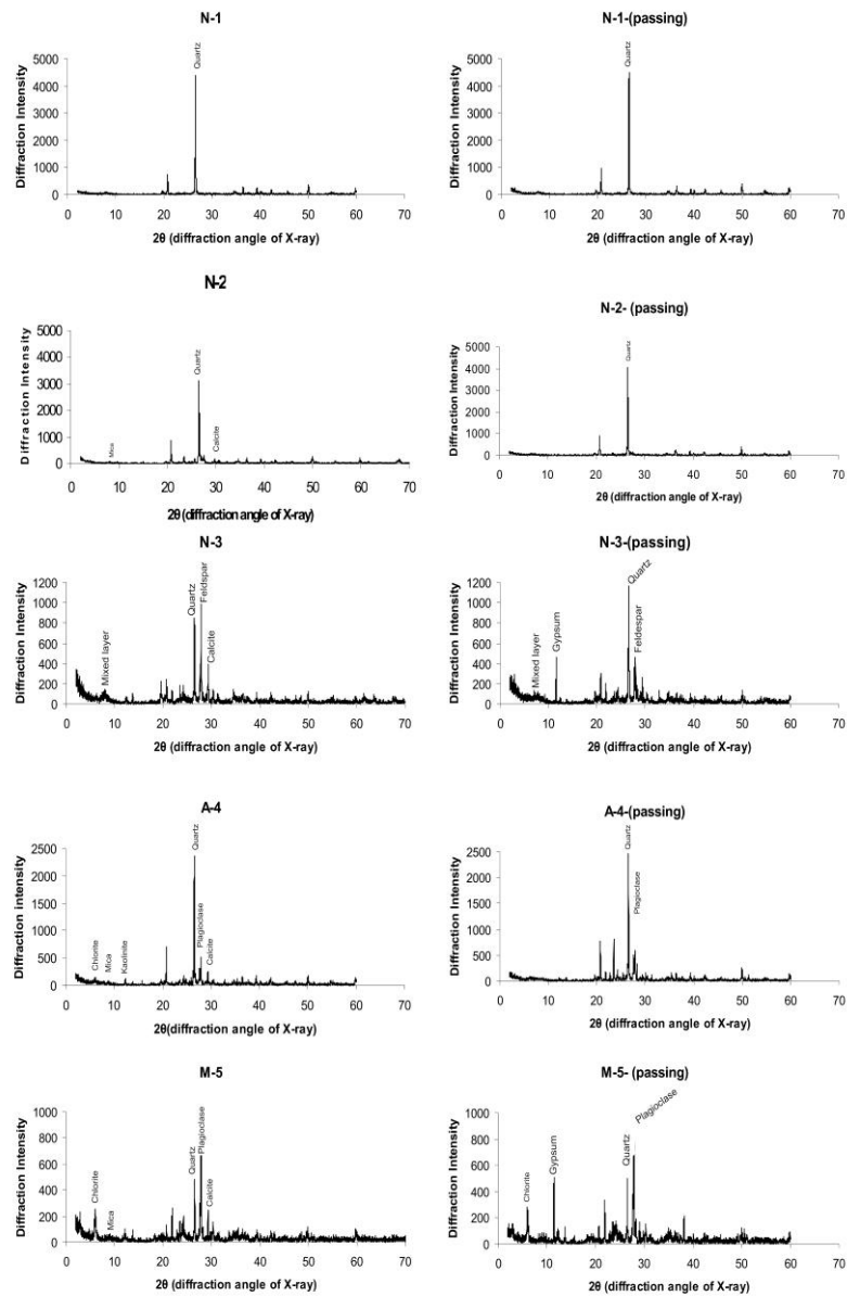
شکل ۴. نتایج آنالیز XRD بر روی نمونه‌های سنگ بکر (نمودارهای سمت چپ) و رسوبات عبور کرده از استوانه مشبک (نمودارهای سمت راست) بعد از انجام ۱۵ سیکل آزمایش دوام و ارتفگی کدهای مربوط در بالای شکل‌ها نشان‌دهنده شماره واحد سنگ‌ها است.
