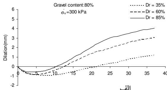
شکل ۱۰. نمودار الف) تنش برشی در مقابل جاب‌جایی افقی،
