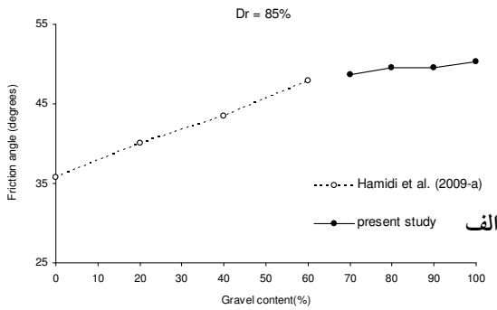
شکل ۱۷. تغییرات زاویه اصطکاک خاک با الف) تراکم نسبی مخلوط
