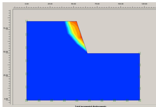
شکل ۳. نمایش تغییرشکل‌های کل برای تحلیل دوبعدی برای ترانشه با ارتفاع ۳۴ متر، شیب ۱ افقی: قائم و مصالح L1-1
