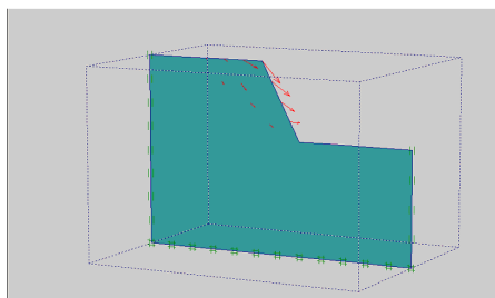
شکل ۳. نمایش تغییرشکل‌های کل برای تحلیل دوبعدی برای ترانشه با ارتفاع ۳۴ متر، شیب ۱ افقی: قائم و مصالح L1-1
