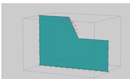
شکل ۳. نمایش تغییرشکل‌های کل برای تحلیل دوبعدی برای ترانسه با ارتفاع ۳۴ متر، شیب ۱ افقی: قائم و مصالح L1-1
