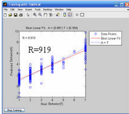
نتایج آموزش شبکه پیش‌بینی رفتار آب‌گذری یا استفاده از ۶ پارامتر
