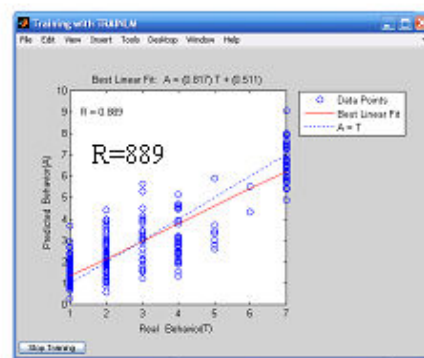
نتایج آموزش شبکه پیش‌بینی رفتار آب‌گذری یا استفاده از ۶ پارامتر و مقدار لوژن
