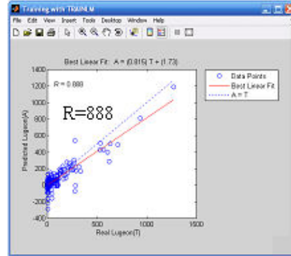
نتایج آموزش شبکه پیش‌بینی مقدار لوژن یا استفاده از ۶ پارامتر
