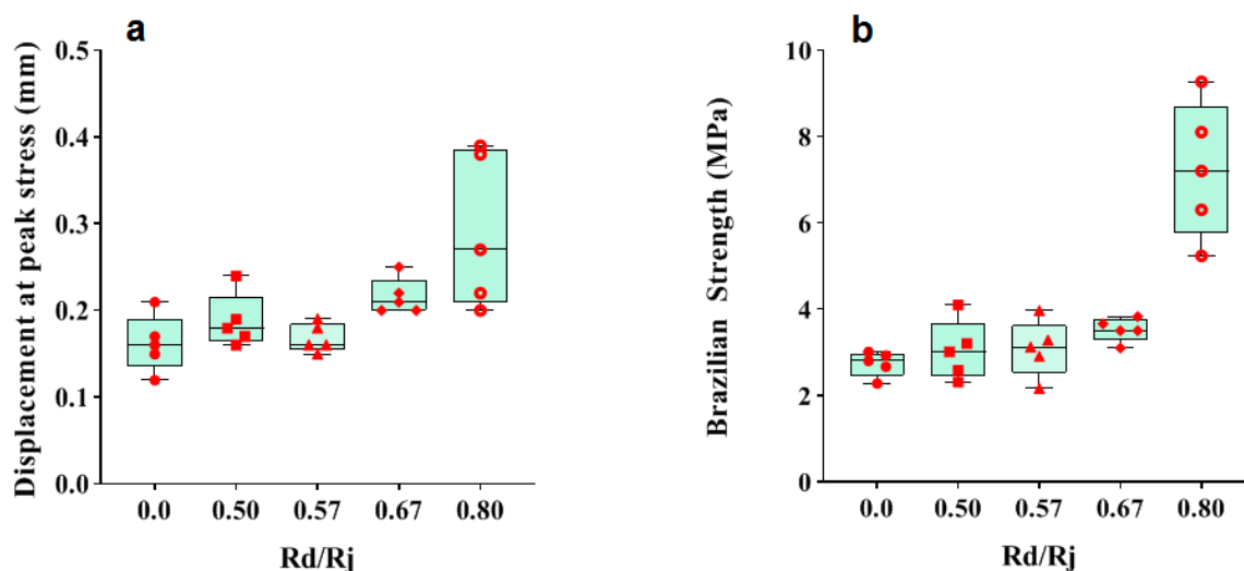
شکل ۶. تأثیر تغییر نسبت شعاع نمونه به شعاع فک ( \rho ) در آزمایش برزلی بر نتایج الف) مقادیر مقاومت کششی تخمین زده، ب) جابه‌جایی متناظر با حداکثر بار
