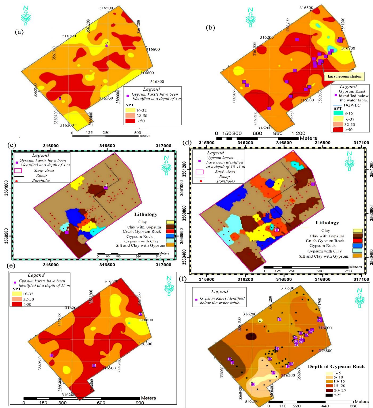
شکل ۱۰. رقومی‌سازی کارست‌های گچی شناسایی شده، (a) در عمق ۴ متری بر روی نقشه پهنه‌بندی مقادیر SPT در عمق ۴/۵ متر، (b) زیر سطح ایستابی بر روی نقشه پهنه‌بندی مقادیر SPT در عمق ۱۰/۵ متر، (c) در عمق ۴ متری بر روی نقشه پهنه‌بندی لیتولوژی مصالح در عمق ۴/۵ متری، (d) در اعماق ۱۰-۱۱ متری بر روی نقشه پهنه‌بندی لیتولوژی مصالح در عمق ۱۰/۵ متری، (e) در عمق ۱۵ متری بر روی نقشه پهنه‌بندی مقادیر SPT در عمق ۱۵ متر و (f) در زیر سطح ایستابی بر روی نقشه پهنه‌بندی سنگ‌بستر محدوده مورد مطالعه Fig. 10. Digitization of gypsum karsts identified, a) at a depth of 4 meters on the SPT zoning map at a depth of 4.5 meters, b) below the water table on the SPT zoning map at a depth of 10.5 m, c) at a depth of 4 meters on a lithology zoning map of materials at a depth of 4.5 meters, d) at depths of 10-11 meters on a lithology zoning map of materials at a depth of 10.5 meters, e) at a depth of 15 meters on the zoning map of SPT values at a depth of 15 meters, and f) below the water table on the bedrock zoning map of the study area.
