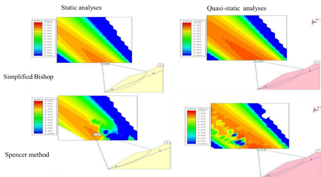
شکل ۱۳. نتایج تحلیل پایداری نرم افزار اسلاید در شرایط اشباع برای پروفیل C Fig. 13. The results of the Slide stability analysis under saturated conditions for profile C
