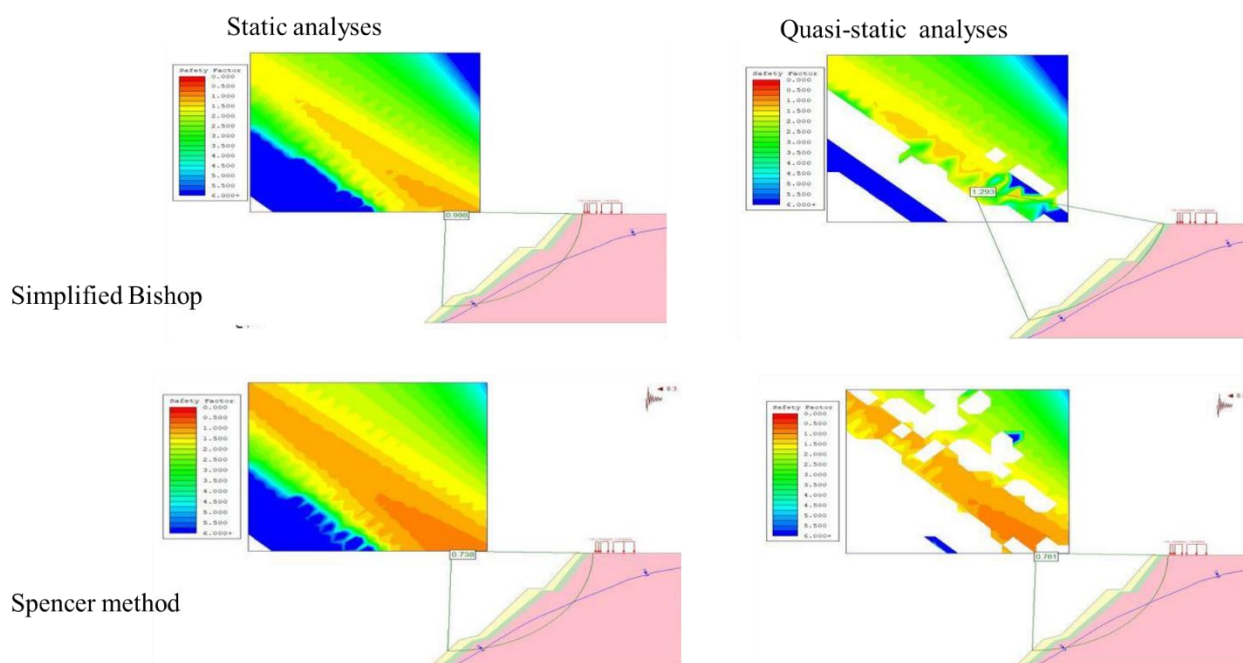
شکل ۱۲. نتایج تحلیل پایداری نرم افزار اسلاید در شرایط اشباع برای پروفیل B Fig. 12. The results of the Slide stability analysis under saturated conditions for profile B
