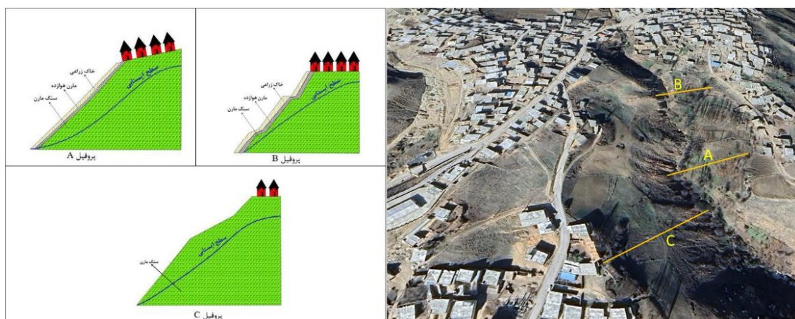
شکل ۸. موقعیت جغرافیایی، وضعیت هندسی و مقاطع زمین‌شناسی پروفیل‌های مورد مطالعه
