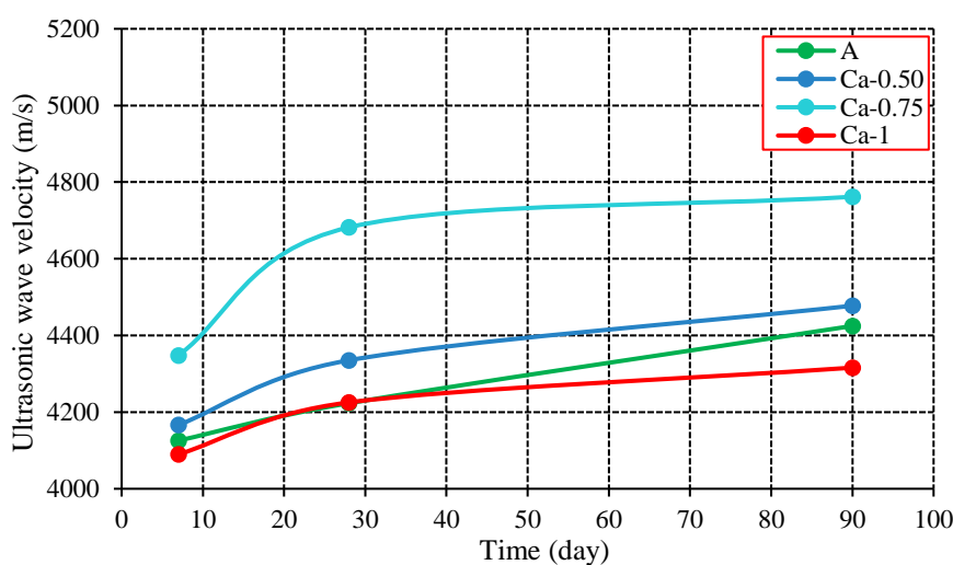
شکل ۱۲. سرعت سیر امواج اولتراسونیک در نمونه‌های حاوی نانوکلسیت
