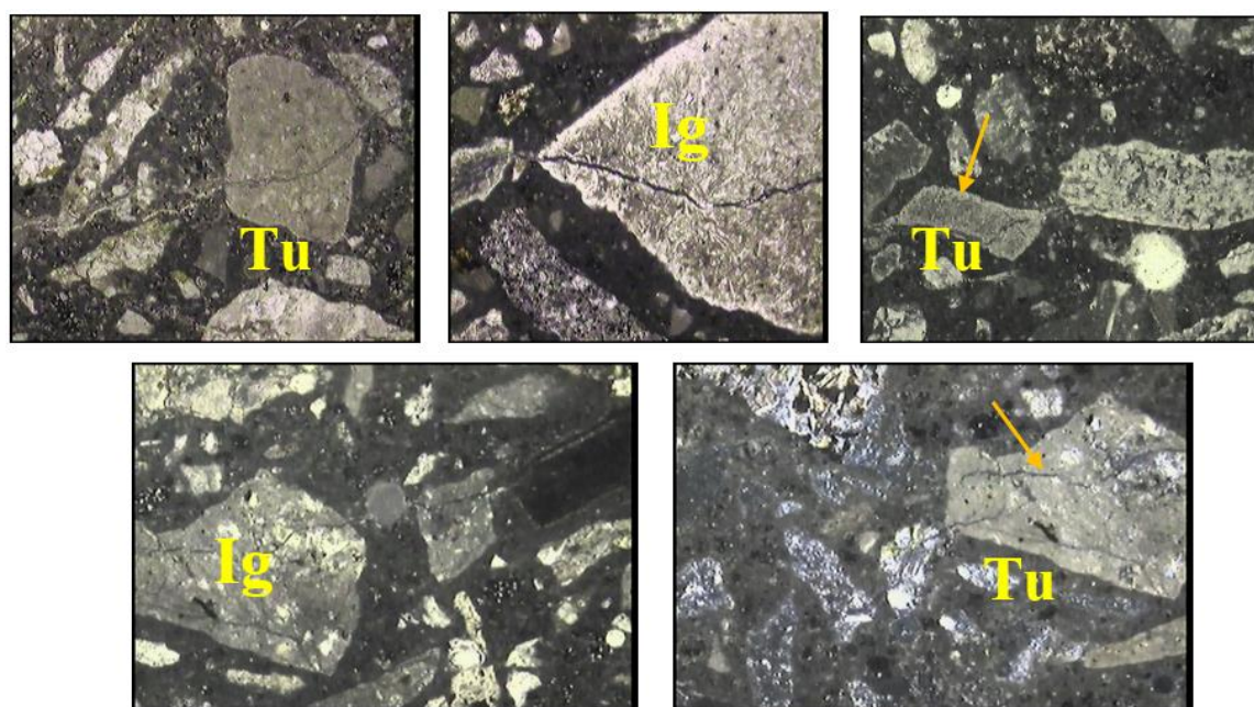
شکل ۱۱. تأیید واکنش قلیایی-سیلیسی سنگدانه‌های بتن توسط آزمایش پتروگرافی بتن و DRI
