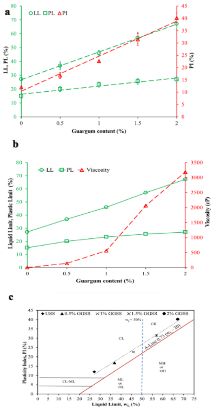
شکل ۱۰. حدود آتربگ خاک بکر و خاک تثبیت شده با صمغ گوار، (a) خواص خمیری (b) حد روانی و حد خمیری در مقابل ویسکوزیته (c) نمودار شاخص پلاستیسیته خاک بکر و گوارگام (Nugent et al., 2009).
