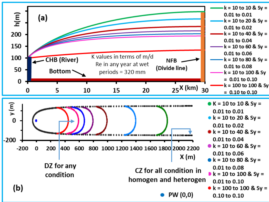
شکل ۹. اثر ناهمگنی: (a) سطح آب نرمال در پایان دوره‌ی تر. (b) حریم آبرفتی و حریم تخلیه. خطوط زمان گذر یک ساله هستند. Fig. 9. The effect of heterogeneity: (a) Normal water level at the end of the wet period. (b) Capture Zone and Discharge Zone. Travel time lines are for 1 year.
