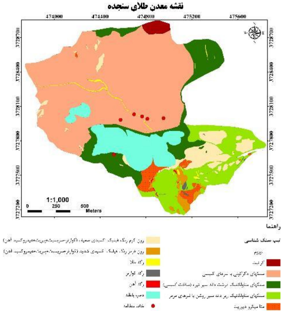
شکل شماره ۲- نقشه زمین شناسی معدن سنجه و محل نمونه‌گیری در شیست‌هایی که در دیواره معدن مشکل ایجاد نموده‌اند [۲۳]
