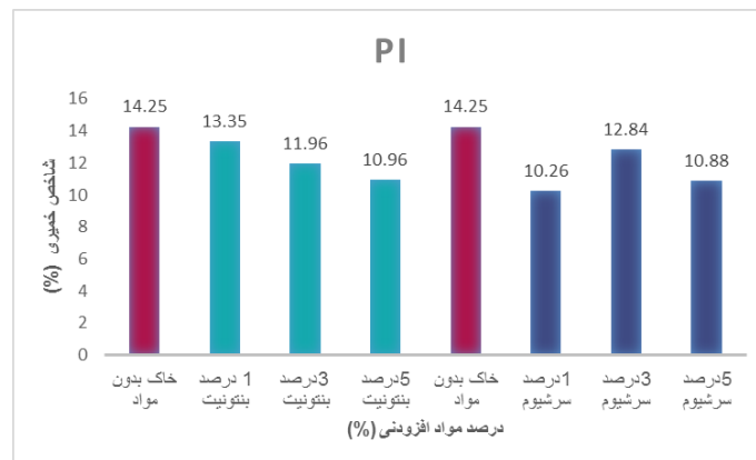
شکل ۴- تأثیر درصدهای وزنی مختلف بنتونیت و سریشوم بر روی شاخص خمیری خاک
